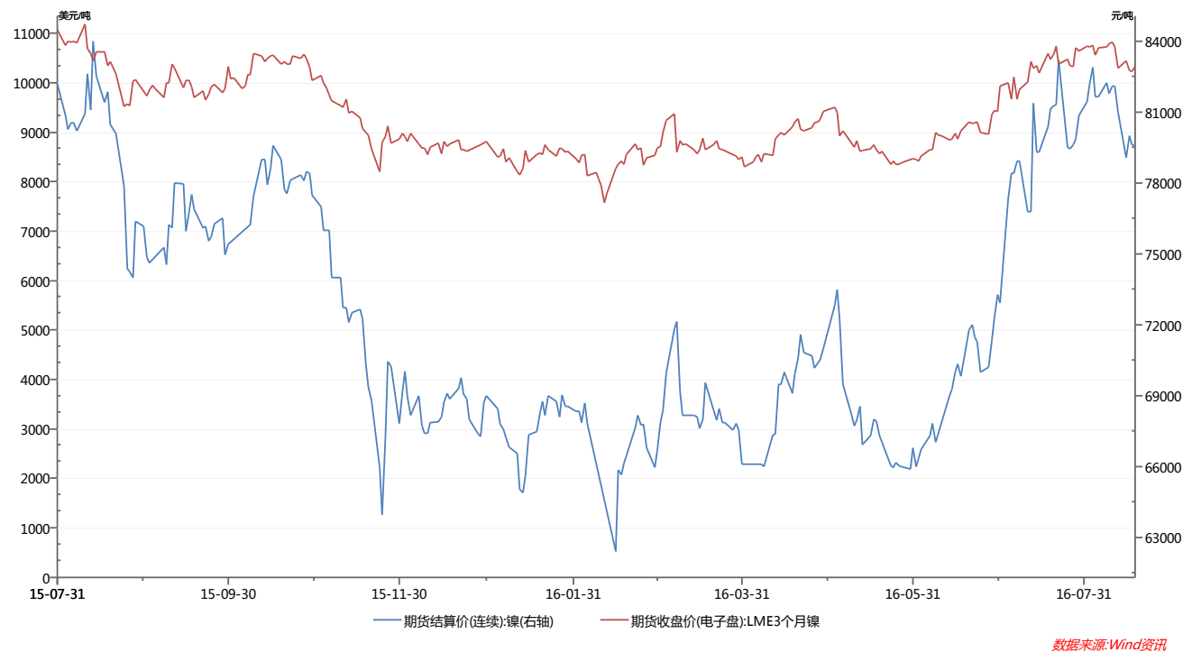
LME3月电子盘及沪镍主力1701（右轴）走势对比
