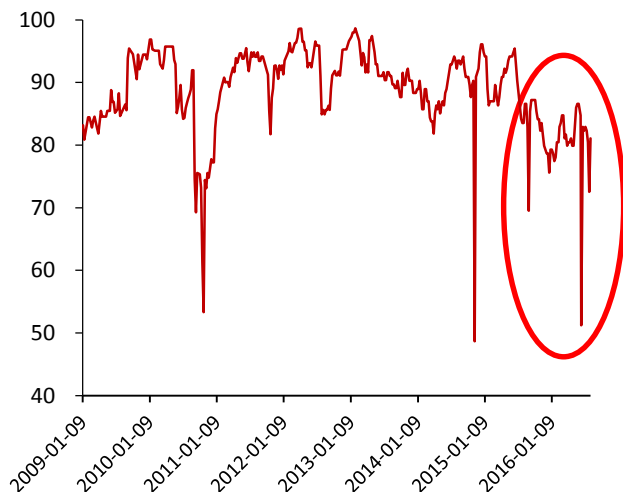
图2：唐山高炉开工率
